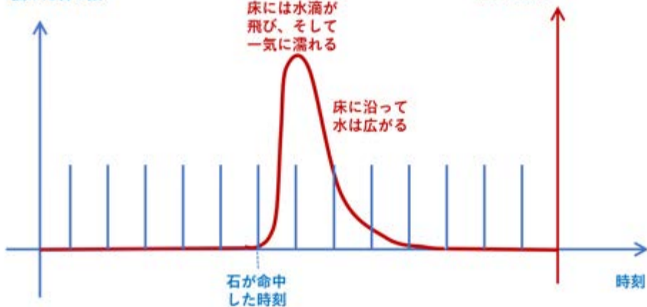
図1：身近な例を考えてわかる、因果関係をデータからとらえることの難しさ
